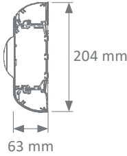
Boitier avec habillage haut et bas
