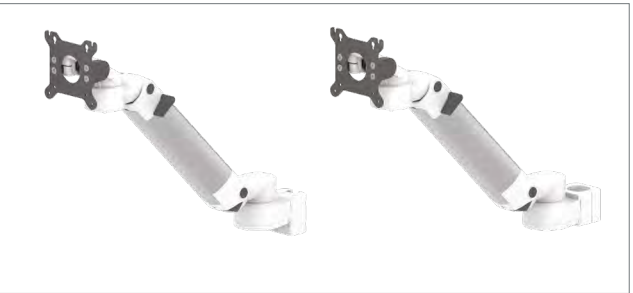
Bras ajustable en hauteur déport de 450 mm, débattement vertical 438 mm pour écran VESA (max 16 kg)
