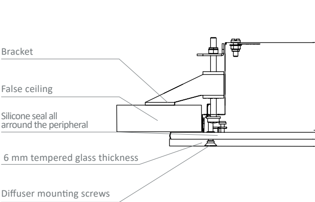
Lay-Out (LO)
