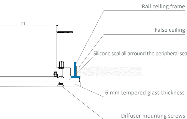
Lay-In (LI)
